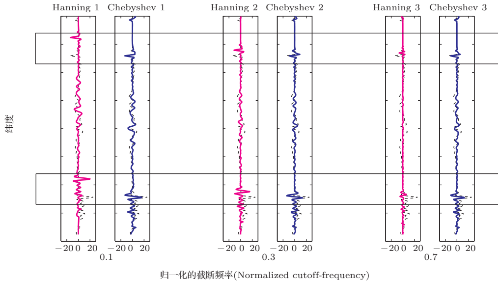
图 4 (网刊彩色) 取三个不同截断频率 (0.1, 0.3, 0.7) 时 170^\circ\text{W} (图 1, 图 2 中白色虚线对应位置) 对应的经向上的流速分布. 黑色虚线为滤波前的流速信号, 粉色为汉宁方法的结果, 蓝色为切比雪夫方法的结果.
